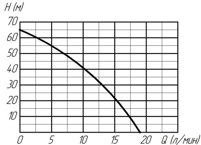
Рисунок 3 – График зависимости показателей напорно-расходных характеристик, H – Напор; Q – Расход.
