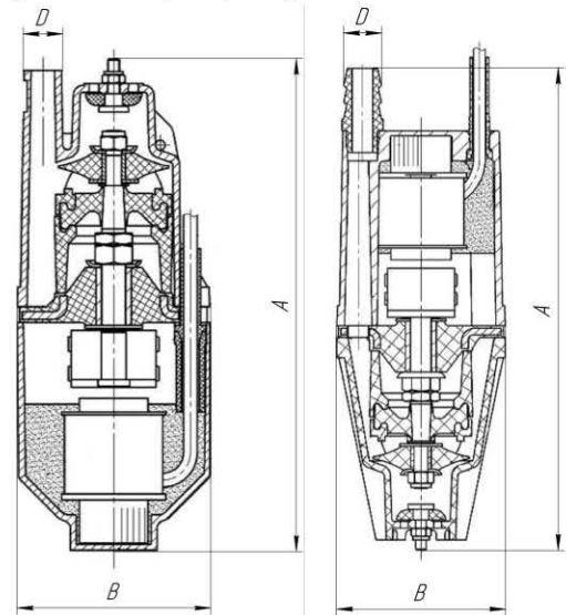
Рисунок 5 – Габаритные и присоединительные размеры изделия
